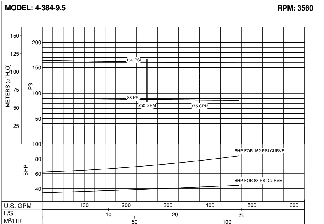
Curve No: PC-219408
