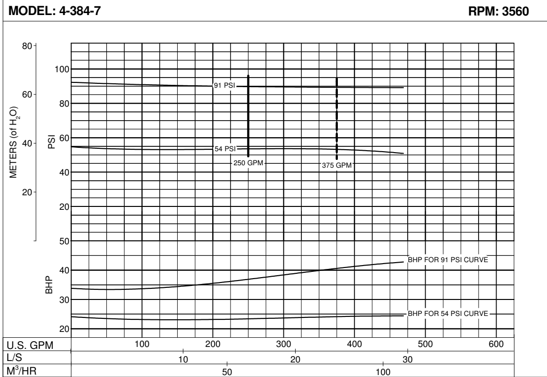
Curve No: PC-219366
